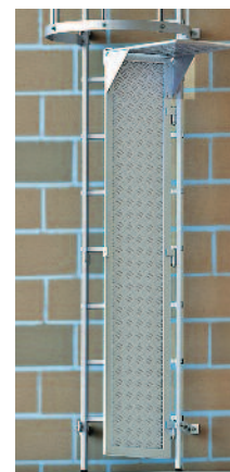
Porte de sécurité avec opercule
